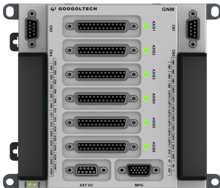
图 1-5 GNM-601-A00 端子板俯视图
