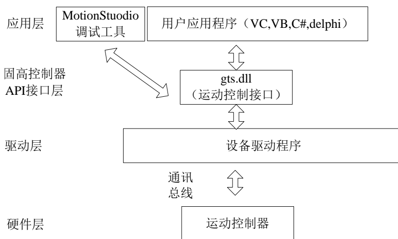
图 2-13 系统架构图
