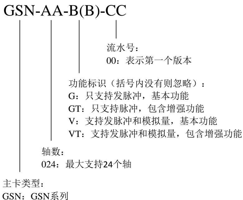
图 1-1 主卡型号说明
