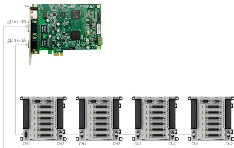
图 2-10 运动控制器与 6 轴端子板连接示意图
