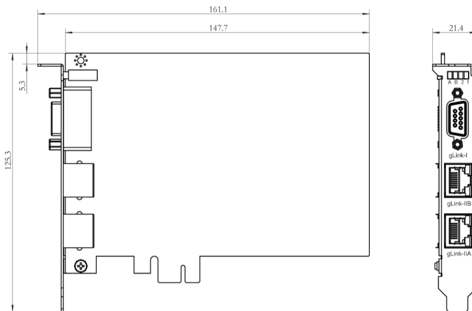
图 1-4 GSN-A00 控制器的侧视图（右）和俯视图
