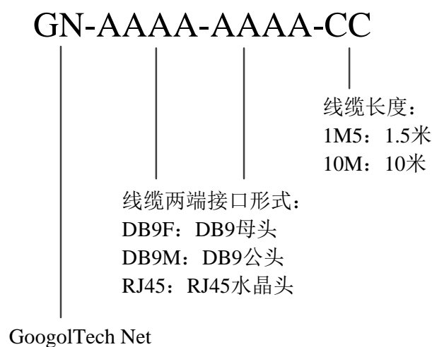
图 1-3 线缆型号说明
