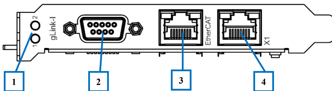
图 1-3 GEN 控制器接口示意图
