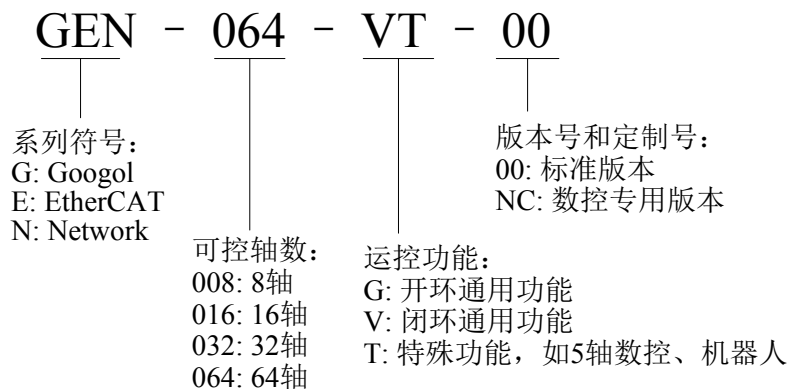
图 1-1 GEN 运动控制器型号说明
